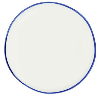
POR056 Dessertteller CLASSIC Ø 16 × 1,5 cm
